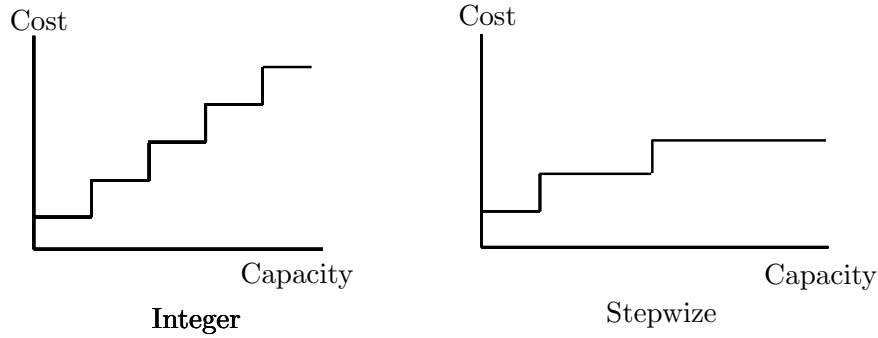
図 3: Cost Function
