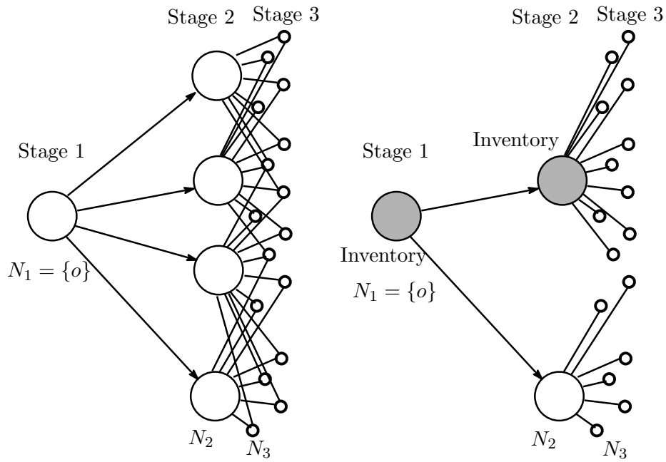
图 1: 3Stage Network
